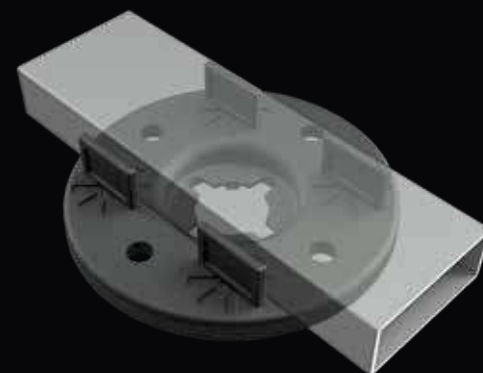
ESEMPIO DI POSA PER PAVIMENTAZIONE DECKING CON SOTTOSTRUTTURA A TRAVETTO (LARGHEZZA MAX 60 MM) EXAMPLE OF LAYING FOR DECKING SYSTEMS WITH JOIST SUPPORT STRUCTURE (WIDTH MAX. 60 MM) EJEMPLO DE COLOCACIÓN PARA SUELOS DE TARIMA CON ESTRUCTURA INFERIOR CON TRAVESAÑOS (ANCHO MÁX. 60 MM)
